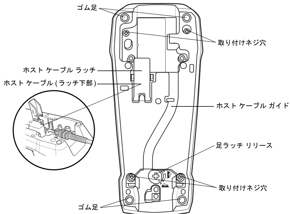
図 1-5 クレードル背面図
